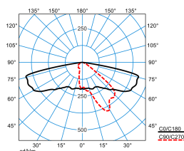
9301K AB2L-LR-SLR3/2900-730 4G3 ET (CLO end value)
