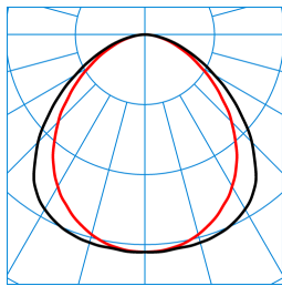
FidescaBS G3 M46 DW19 30-840 ETDD TX774416
