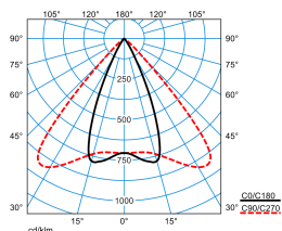
E-Line PRO 78 Grado WRS-DF84 40-840 M43 ET 05 05
