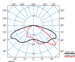
LnPlus 40-AB7L-SLR1/6200-722 6G1 ET (CLO end value)
