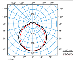
Olisq LWD2 DW 40-840 ETBLE +CAS-S IP54
