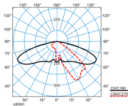
Publisca P2-AB2L-LRA/3800-730 6G1S TX047796 DIN 5040: A30 UTE: 1,00 G DLOR: 100 % ULOR: 0 % CEN Flux Code: 35 74 97 100 100
