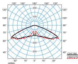
Publisca P1W-RB6L-LR/1200-730 2G1S ET (CLO initial value)
