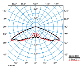
Publisca P1W-RB6L-LR/1200-730 2G1S ET (CLO end value)
