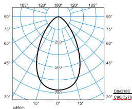
E-Line PRO 78IP50 MironaF TB 200-840 ETDD L150 01 ESG 01 IP50 (LEO2)
