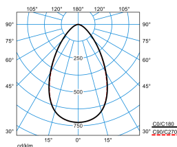
E-Line PRO 78IP50 MironaF TB 200-840 ETDD L150 01 ESG 01 IP50 (LEO1)
