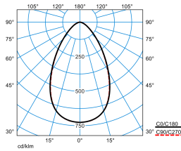
E-Line PRO 78IP50 MironaF TB 200-840 ETDD L150 01 ESG 01 (LEO2)
