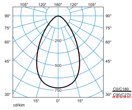
E-Line PRO 78IP50 MironaF TB 270-840 ET L225 01 ESG 01 IP50 (LEO1)
