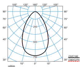
E-Line PRO 78IP50 MironaF TB 270-840 ET L225 01 ESG 01 IP50 (LEO2)
