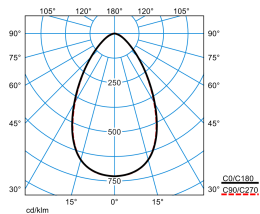
E-Line PRO 78IP50 MironaF TB 270-840 ET L225 01 ESG 01 (LEO3)
