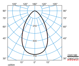
E-Line PRO 78IP50 MironaF TB 270-840 ET L225 01 ESG 01 (LEO2)
