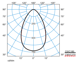
E-Line PRO 78IP50 MironaF TB 270-840 ET L225 01 ESG 01 (LEO1)
