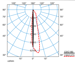
Skeo Q-W2 GT AE2R/70-840 ETDD
