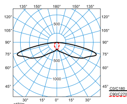
LIQ 50N-SB3L-SLR1/2200-740 2G1 ET (CLO end value)
