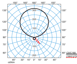
Luceos S-T G3 PAW-IL 300-840 ETDS 03 (LEO2)
