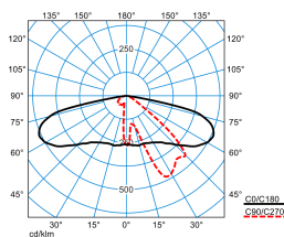
Publisca P1-AB2L/1100-740 2G1S ETDD (CLO initial value)
