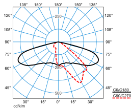
Jovie 50-AB2L6S3-34-7TW-ET-CAB-26 (DSU-CLO initial value)
