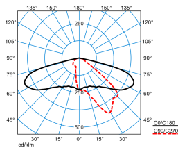
Jovie 50-AB2L6S3-34-7TW-ET-CAB-26 (DWW-CLO end value)
