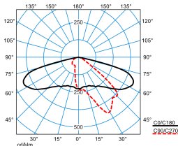
Jovie 50-AB2L6S3-34-7TW-ET-CAB-26 (DCW-CLO end value)
