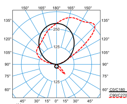
Luceos S G3 PAW-IA 170-9TW ETDI KL 01 (DSU)
