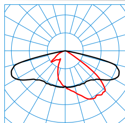
LIQ 70N-AB7L-LR/10000-727 12G1 ET(CLO end value) TX278264 ■ C0 - C180 ■ C90 - C270 DIN 5040: A30 UTE: 1,00 E DLOR: 100 % ULOR: 0 % CEN Flux Code: 39 76 98 100 100
