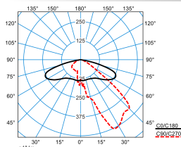
Publisca P2-AB2L-LR/3500-730 4G1S TX047757 DIN 5040: A30 UTE: 1,00 G DLOR: 100 % ULOR: 0 % CEN Flux Code: 35 73 97 100 100
