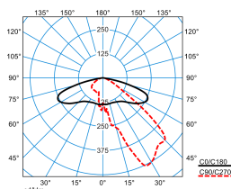
Publisca P2-AB2L-LR/3500-730 4G1S ET (CLO end value) TX301557 DIN 5040: A30 UTE: 1,00 G DLOR: 100 % ULOR: 0 % CEN Flux Code: 35 73 97 100 100
