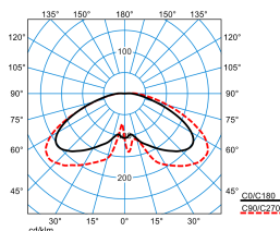
Publisca P1W-RBT-LRA/2600-740 3G1S ET (CLO end value)
