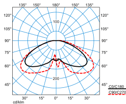
Publisca P1W-RBT-LRA/2600-740 3G1S ET (CLO initial value)
