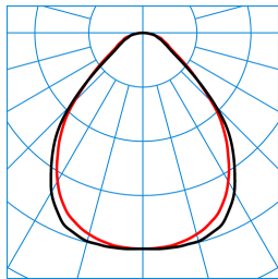
ArimoFit G2 M84 PW19 42-940 ETDD + ArimoFit G2 Sky M84-TS ZER TX427385
