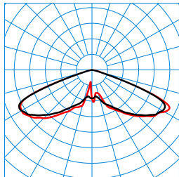
Publisca P1-RB6L-LRA/2600-730 3G1S ET (CLO end value) TX301711 ■ C0 - C180 ■ C90 - C270 DIN 5040: A20 UTE: 1,00 J DLOR: 100 % ULOR: 0 % CEN Flux Code: 20 57 98 100 100
