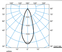
CPL G2 3P FL 30-830 M33 ET L1,5 05
