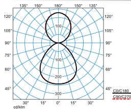
Lunexo H2 CDP-I 8800 830 ETDD 03 TX774007
