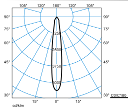
E-Line PRO 78 BV G2 RF-SP 40-840 M35 ET 01 Blank
