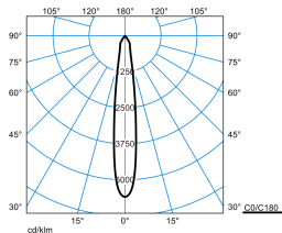
E-Line PRO 78 BV G2 RF-SP 40-840 M35 ET 01 01
