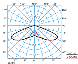
Publisca P2-RB6L/1100-740 2G1S
