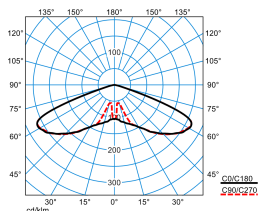
Publisca P1-RB6L/1000-740 2G1S ETDD (CLO end value)
