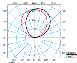
Sanesca W2 4600-8TW ETDD/ET 830 01 (DSU)
