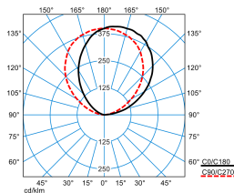
Sanesca W2 4600-8TW ETDD/ET 830 01 (DCW)
