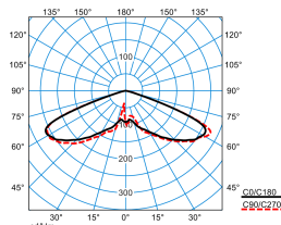
Publisca P1-RB6L-LR/2000-730 3G1S
