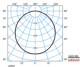
Olisq QWD3 DW 30-840 ETBLE +CAS-S IP54 + Olisq QWD3 ZDR 1/1 01
