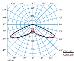
Publisca P1W-RB6L-LR/3800-730 6G1S ET (CLO initial value)
