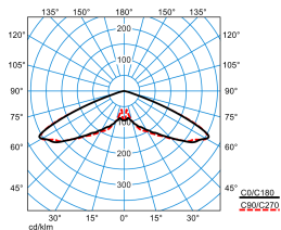
Publisca P1W-RB6L-LR/3800-730 6G1S ET (CLO end value)
