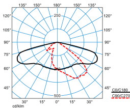
LnPlus 60-AB7L-LR/26000-722 24G1 ET (CLO end value) TX390198
