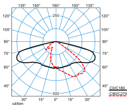
LnPlus 60-AB7L-LR/26000-722 24G1 ET (CLO initial value) TX390182
