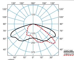
LnPlus 40-AB7L-SLR2/10000-740 8G1 ET (CLO initial value)
