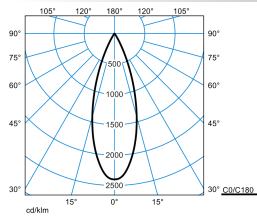
7651 LentyP L-FL 20-BF M54 ET 05 (150) TX781438
