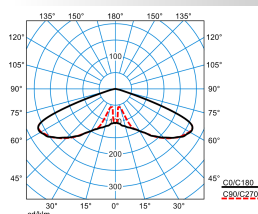
Publisca P2-RB6L/1800-740 2G1S
