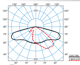
LIQ 90-AB7L-SLR2/29000-740 24G1S ET
