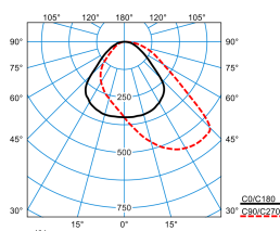
Cultega T COM PAW 600-9TW ETDI KL 01 (DSU)
