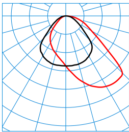
Cultega T COM PAW 600-9TW ETDI KL 01 (DWW) TX875497 ■ C0 - C180 ■ C90 - C270 DIN 5040: A40 UTE: 1.00 D DLOR: 100 % ULOR: 0 % CEN Flux Code: 54 85 97 100 100
