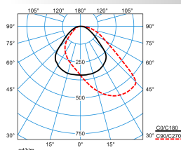
Cultega T COM PAW 600-9TW ETDI KL 01 (DWW)
