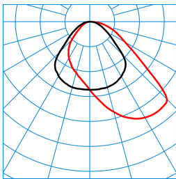
Cultega T COM PAW 600-9TW ETDI KL 01 (DSU) TX875482 ■ C0 - C180 ■ C90 - C270 DIN 5040: A40 UTE: 1.00 D DLOR: 100 % ULOR: 0 % CEN Flux Code: 54 85 97 100 100
