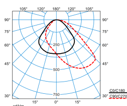
Cultega T COM PAW 600-9TW ETDI KL 01 (DCW)
