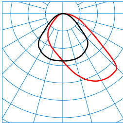
Cultega T COM PAW 600-9TW ETDI KL 01 (DCW) TX875489 ■ C0 - C180 ■ C90 - C270 DIN 5040: A40 UTE: 1.00 D DLOR: 100 % ULOR: 0 % CEN Flux Code: 54 85 97 100 100
