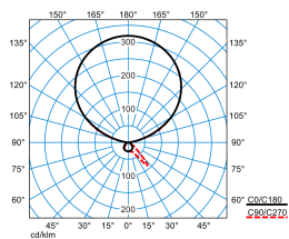
Luceos S-U G3 PAW-IL 300-9TW ETDI 03 (DCW) (LEO1)
