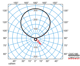
Luceos S-U G3 PAW-IL 300-9TW ETDI 03 (DWW) (LEO1)
