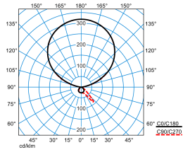
Luceos S-U G3 PAW-IL 300-9TW ETDI 03 (DWW) (LEO2)
