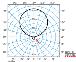
Luceos S-U G3 PAW-IL 300-9TW ETDI 03 (DSU) (LEO2)
