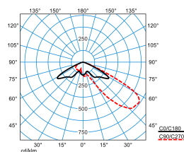
LnPlus 40-AM19L/13500-722 12G1 ETDD (CLO end value)
