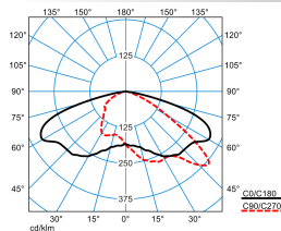
LnPlus 40-AB7L-SLR2/8200-730 8G1 ET (CLO initial value)
