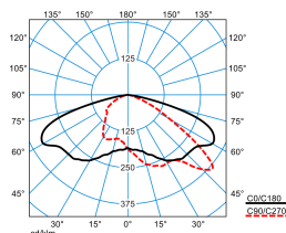
LnPlus 40-AB7L-SLR2/8200-730 8G1 ET (CLO end value)
