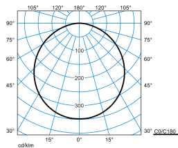
Olisq RWD2 DW 40-840 ET EB3 PC + Olisq RWD2 ZDR 1/1 05
