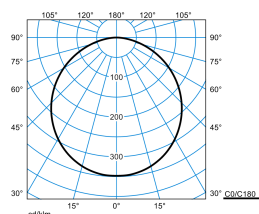
Olisq RWD2 DW 40-840 ET EB3 PC + Olisq RWD2 ZDR 1/1 01
