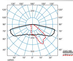
9301K AB2L-LR-SLR3/3500-740 4G3 ET (CLO initial value)
