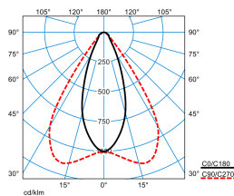
E-Line PRO 78IP50 MironaF HR 270-840 ETDD L225 01 ESG Blank (LEO3)
