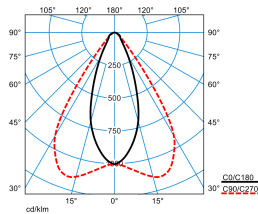
E-Line PRO 78IP50 MironaF HR 270-840 ETDD L150 01 ESG Blank IP50 (LEO1)
