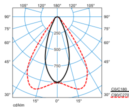
E-Line PRO 78IP50 MironaF HR 270-840 ETDD L150 01 ESG Blank IP50 (LEO2)
