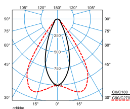
E-Line PRO 78IP50 MironaF HR 270-840 ETDD L225 01 ESG Blank (LEO2)
