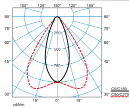
E-Line PRO 78IP50 MironaF HR 270-840 ETDD L225 01 ESG Blank (LEO1)
