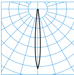
Inveria C 150 RE7R/2200-830 1G1P ET TX460574 ■ C0 - C180
