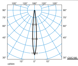
Inveria C 150 RE7R/2200-830 1G1P ET
