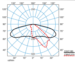
Jovie 50-AB2L-2-10-730-CLO-B
