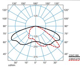
Jovie 70-AB7L-18-180-730-CLO-B
