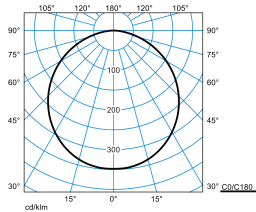
Olisq RWD3 DW 30-840 ET EB3 PC + Olisq RWD3 ZDR 1/1 05
