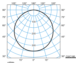
Olisq RWD3 DW 30-840 ET EB3 PC + Olisq RWD3 ZDR 1/1 03
