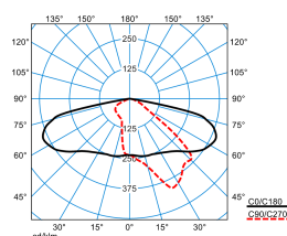
LIQ50N-AB2L6S3-34-7TW-ET-CAB-26 (DSU-CLO end value)
