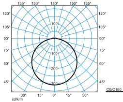
Olisq RWD2 DW 40-830 ET IP54 PC + Olisq RWD2 C 01
