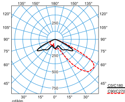
LnPlus 70-AM19L-LR/42000-722 36G1 ET (CLO initial value)
