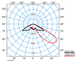
LnPlus 70-AM19L-LR/42000-722 36G1 ET (CLO end value)
