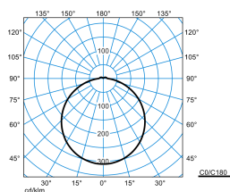
Olisq RWD2 DW 14-40/4/ML-840 IP54 ET + Olisq RWD2 C 01 (stage 1)
