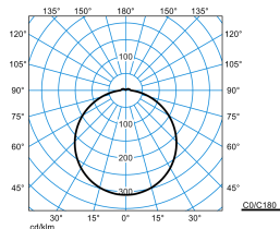
Olisq RWD2 DW 14-40/4/ML-840 IP54 ET + Olisq RWD2 C 01 (stage 4)
