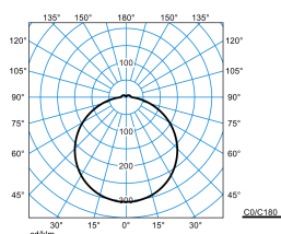
Olisq RWD2 DW 14-40/4/ML-840 IP54 ET + Olisq RWD2 ZDR 1/2 03 (stage 2)
