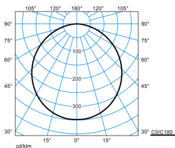
Olisq RWD2 DW 14-40/4/ML-840 IP54 ET + Olisq RWD2 ZDR 1/1 05 (stage 3)
