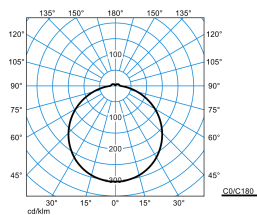
Olisq RWD2 DW 14-40/4/ML-840 IP54 ET + Olisq RWD2 ZDR 1/2 03 (stage 4)
