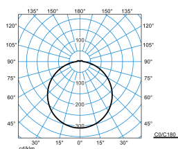
Olisq RWD2 DW 14-40/4/ML-840 IP54 ET + Olisq RWD2 C 01 (stage 2)
