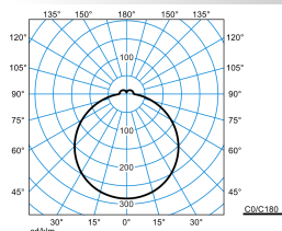
Olisq RWD2 DW 14-40/4/ML-840 IP54 ET (stage 1)
