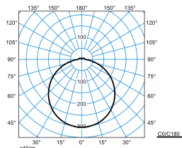
Olisq RWD2 DW 14-40/4/ML-840 IP54 ET + Olisq RWD2 ZDR 1/2 05 (stage 4)
