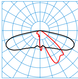
Publisca P2-AB2L/2400-740 3G1S TX047713 ■ C0 - C180 ■ C90 - C270 DIN 5040: A30 UTE: 1,00 l DLOR: 100 % ULOR: 0 % CEN Flux Code: 34 71 96 100 100
